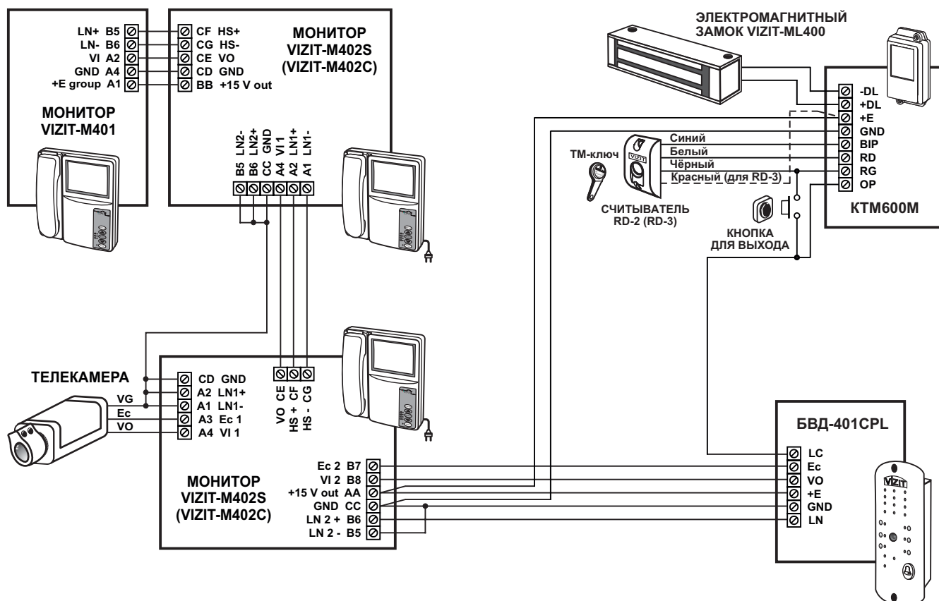
Рисунок 3 - Схема соединений БВД-401CPL с мониторами VIZIT-M401 , VIZIT-M402S (VIZIT-M402C) , контроллером VIZIT-KTM600M и электромагнитным замком VIZIT-ML400
