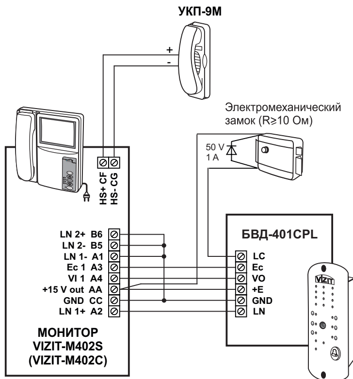
Рисунок 6 - Схема соединений БВД-401CPL с монитором VIZIT-M402S (VIZIT-M402C) и УКП-9М
